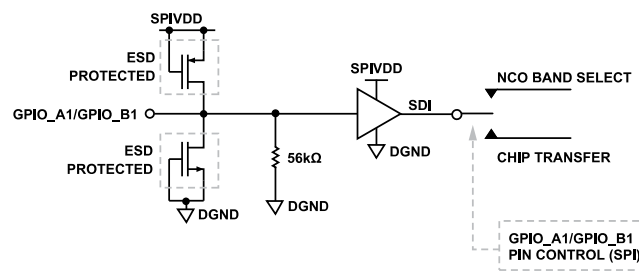
Figure 52. GPIO_A1/GPIO_B1
