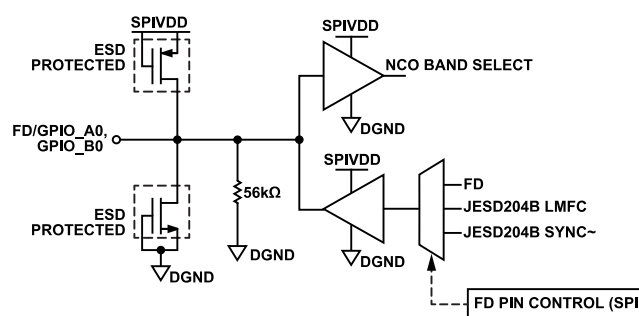
Figure 51. FD/GPIO_A0, GPIO_B0
