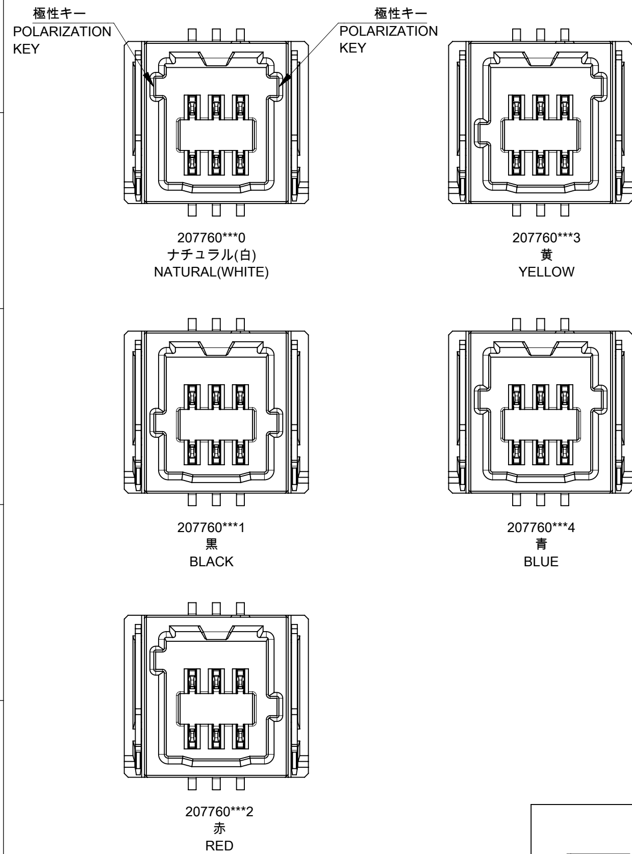
カラー & キー位置 (4,6極) COLOR & KEY POSITION (4,6 CIRCUIT)
