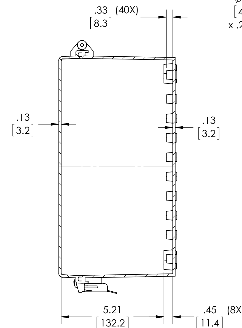
SECTION A-A SCALE 1 : 3
