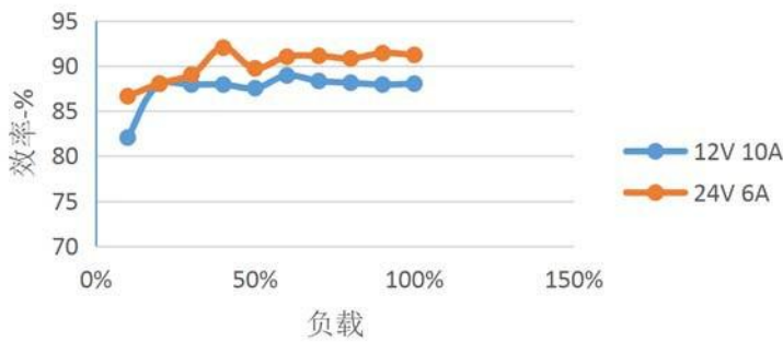
效率VS负载曲线
