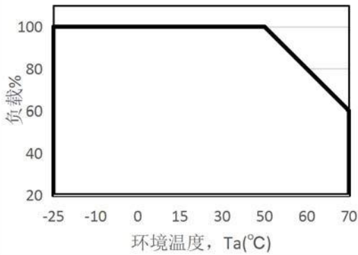
输出负载VS环境温度
