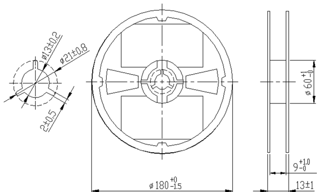
Reel Dimensions
