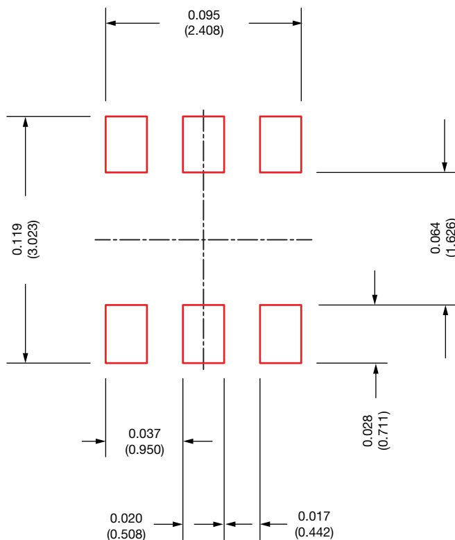
TSOP-5L
