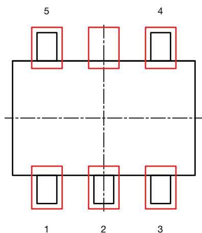
TSOP-5L
