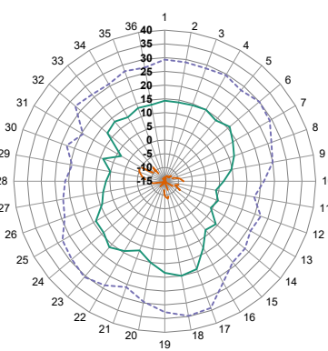
YZ-Plane Gain
