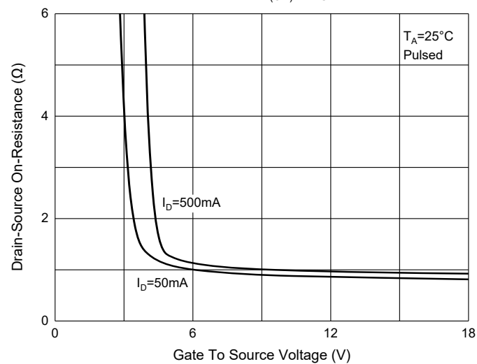
Fig. 3 - R_{DS(ON)} - V_{GS}
