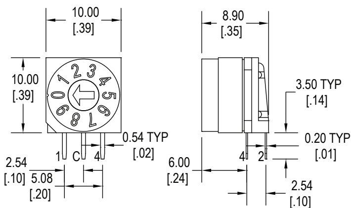
VA Terminals
