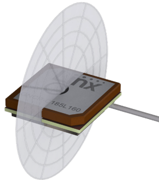
YZ-Plane Gain
