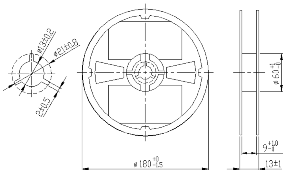
Reel Dimensions
