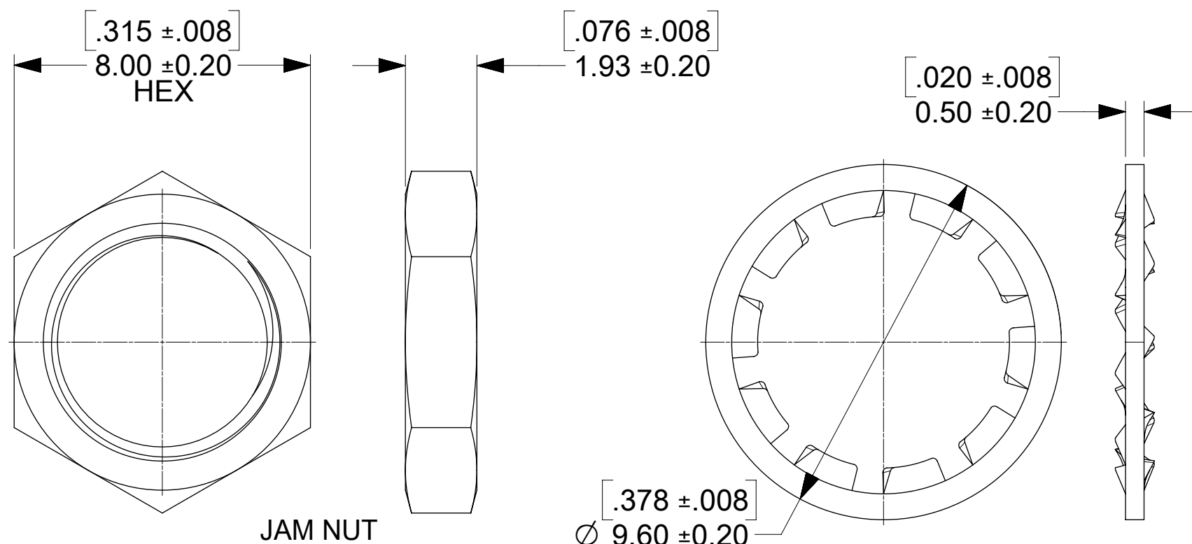
LOCKWASHER
