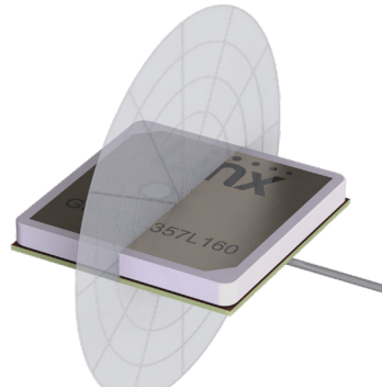
YZ-Plane Gain
