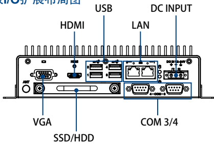
前面板I/O扩展布局图
