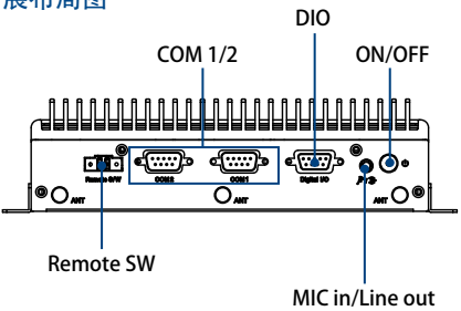
后面板I/O扩展布局图
