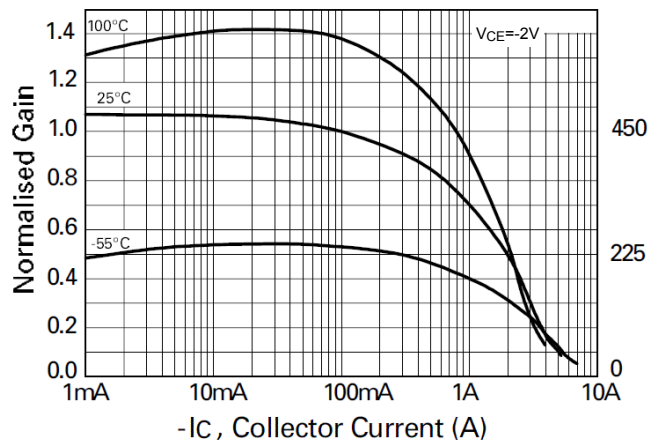
h_{FE} \vee I_C
