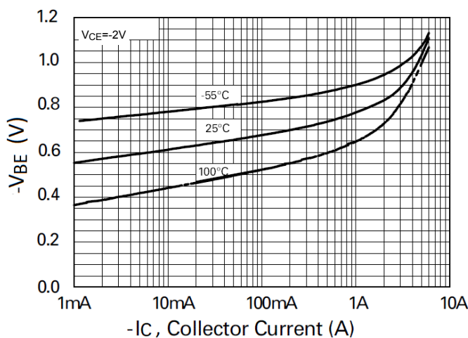
V_{BE(on)} \vee I_C
