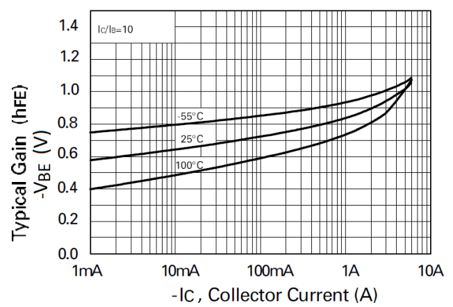
V_{BE(sat)} \vee I_C
