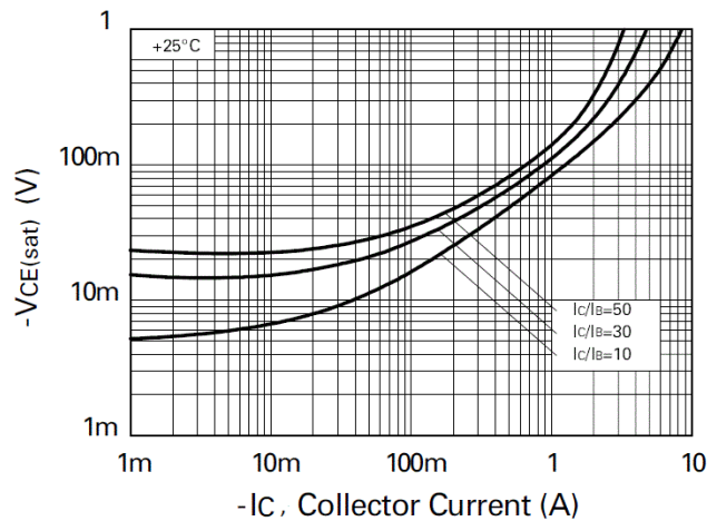
V_{CE(sat)} \vee I_C
