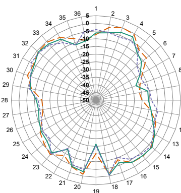
XZ-Plane Gain
