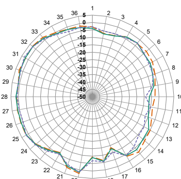
XZ-Plane Gain
