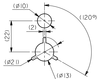
DETAIL Y
