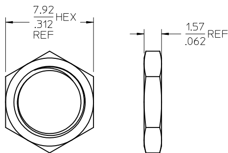
JAM NUT
