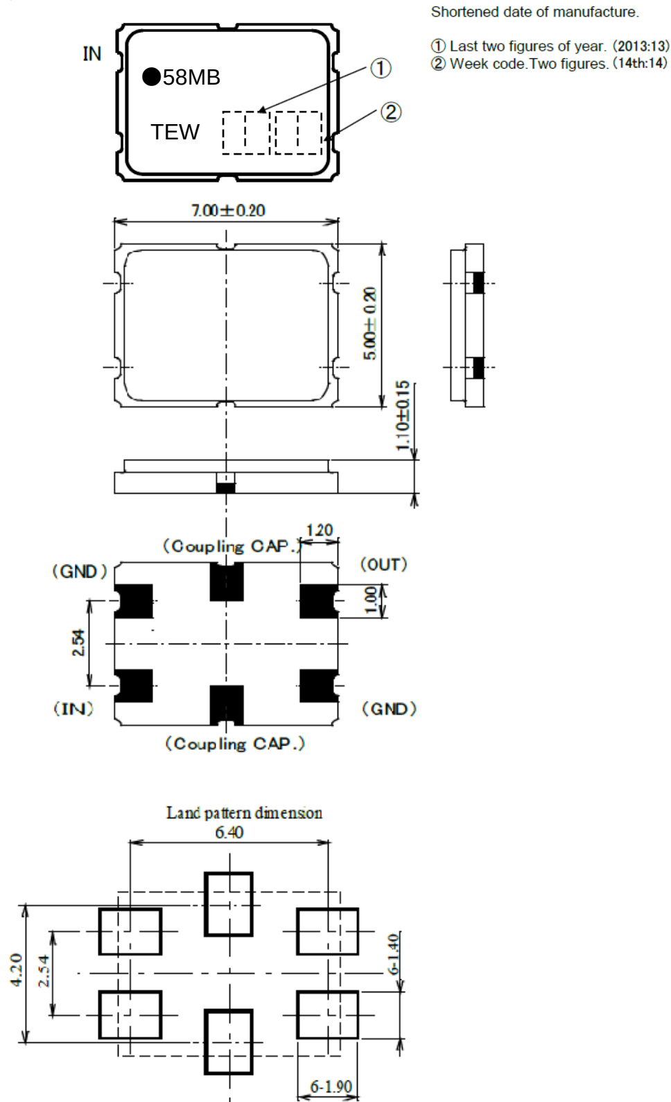
第1図 外形寸法図 Figure 1.Dimensions
