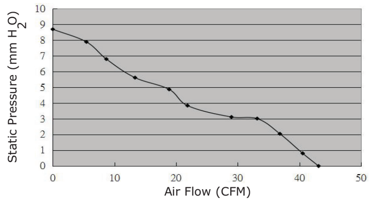
CFM-7025B-240-394
