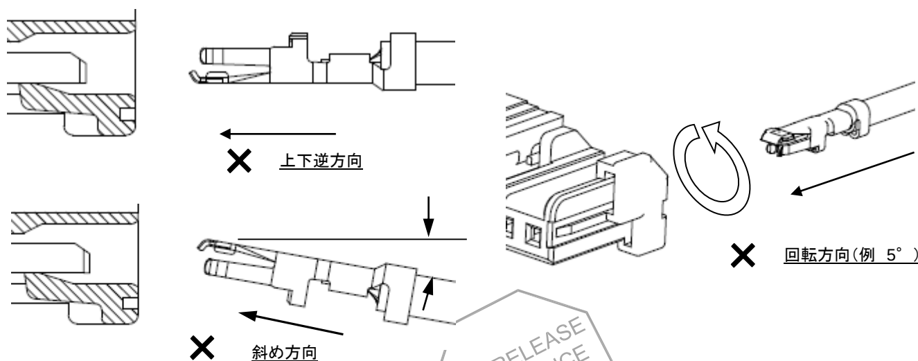
Fig.6-3 不適切な装着方向
