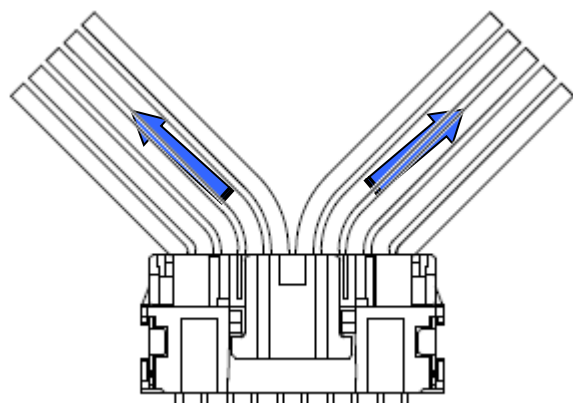
Fig.9-3-3 2方向以上の電線引き回し状態
