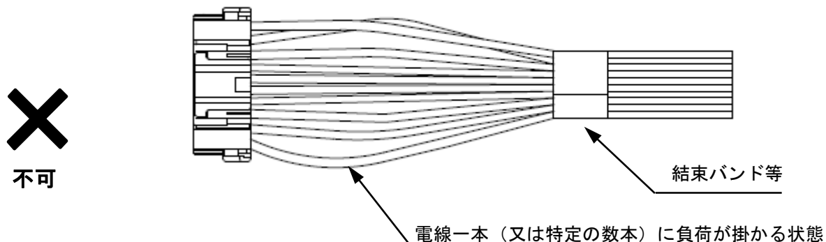
Fig.7-2 不適切なハーネス結束状態
