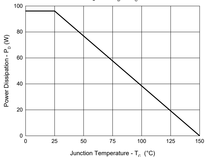
Fig. 10 - P_D - T_C
