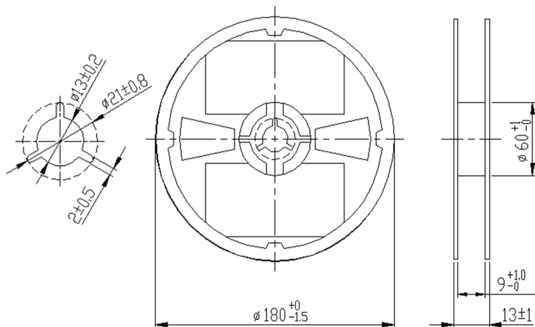
Reel Dimensions
